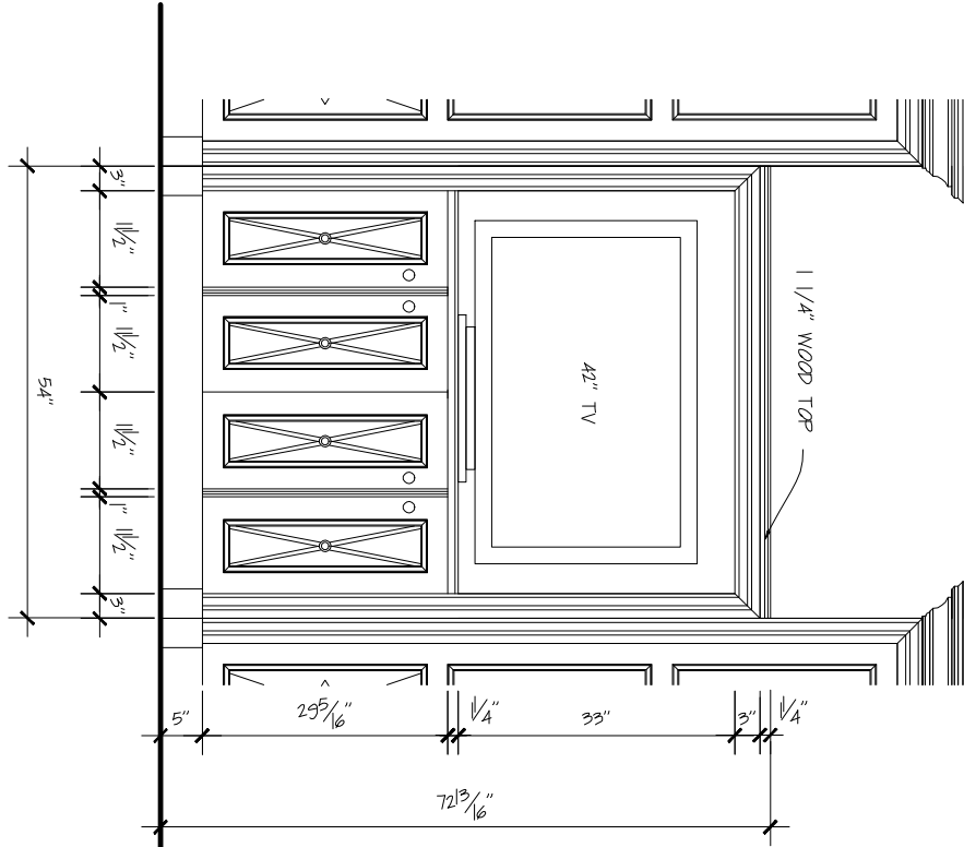
ELEVATION B
